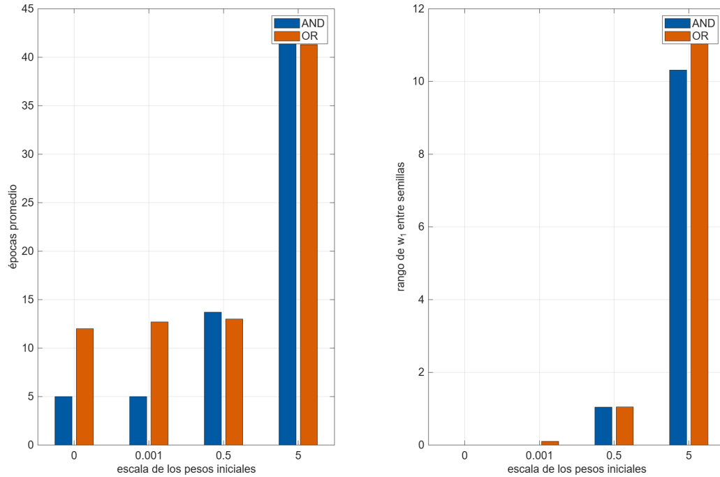
Figura 2: Efecto de la escala de los pesos iniciales en el Perceptrón con la regla 3. A la izquierda las épocas promedio hasta converger y a la derecha la dispersión de los pesos finales entre semillas
